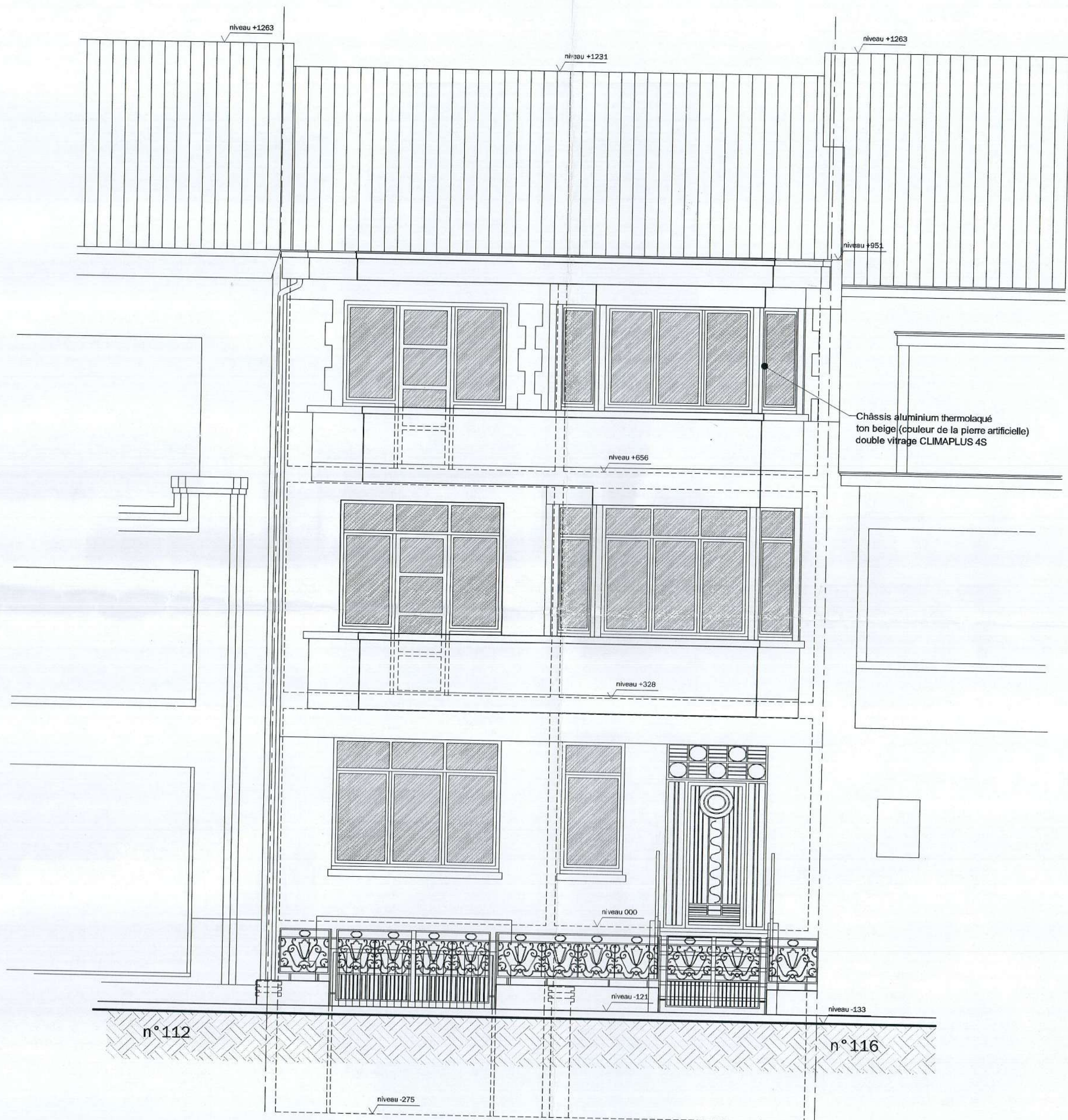
Façade avant (Avenue des Cerisiers n°114)
