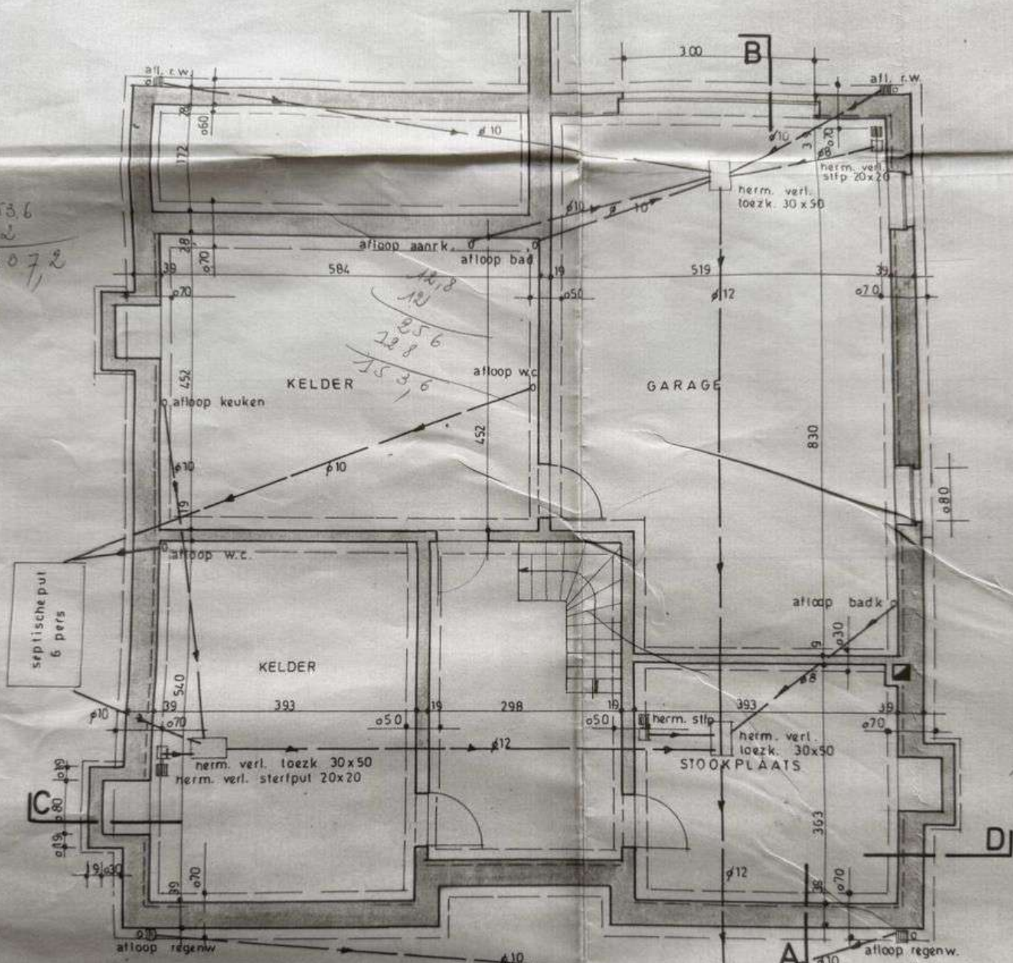
kelder - funderings & rioleringsplan.
