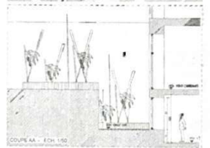
COUPE AA - ECH 1/50
