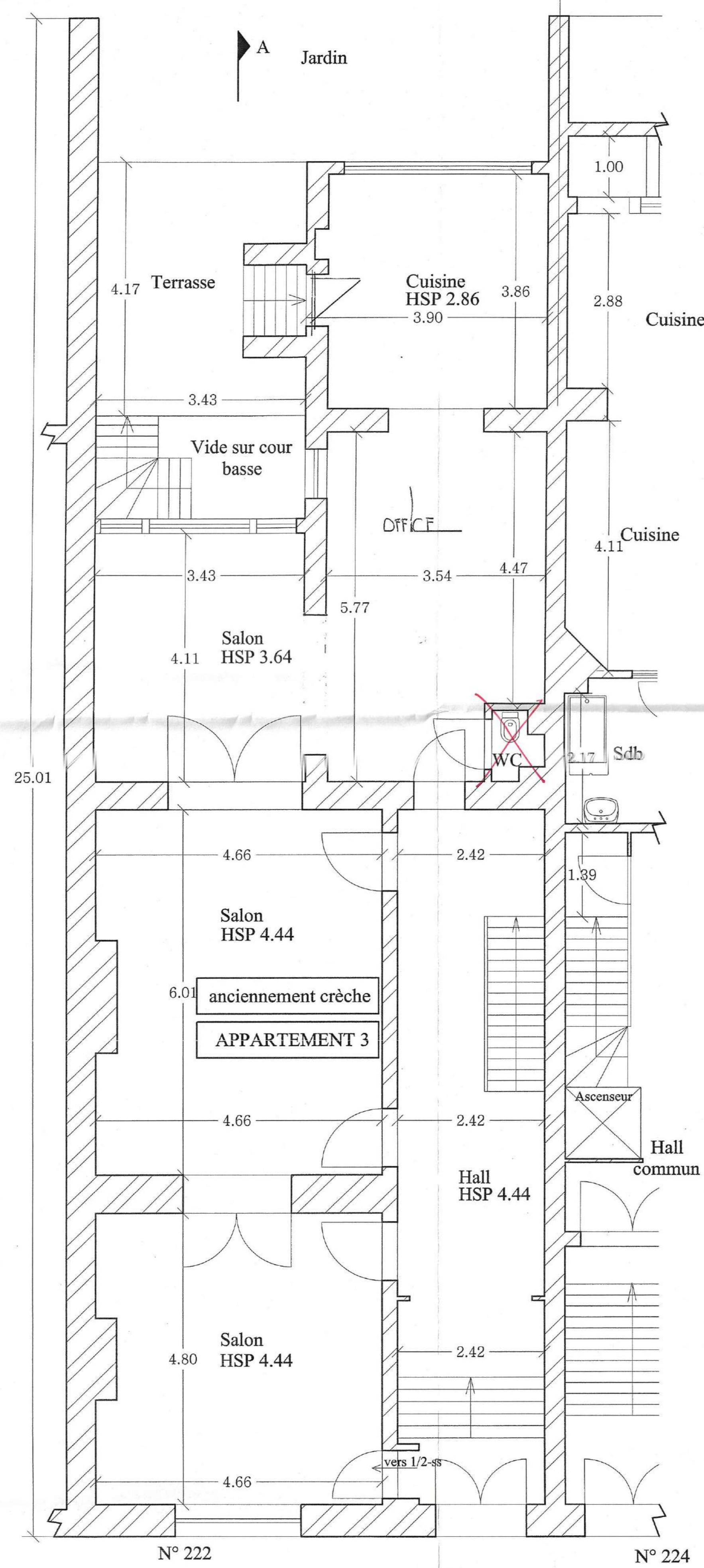
PLAN REZ DE CHAUSSEE
