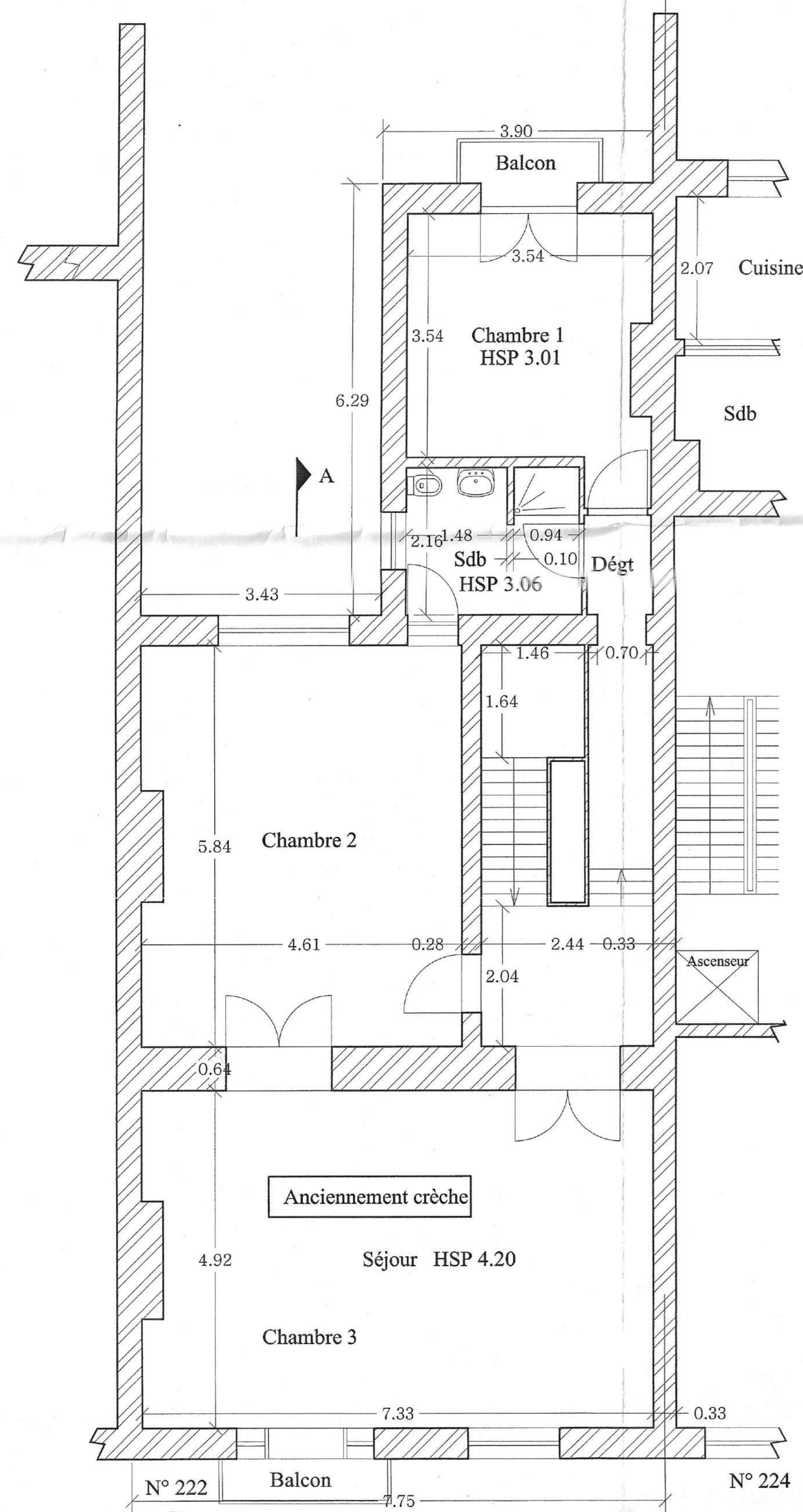
PLAN 1ER ETAGE
