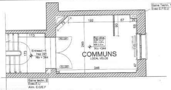
ENTRESOL +1 situation projetée
