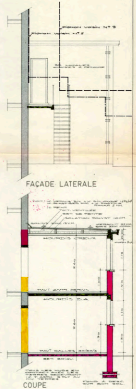
COUPE
