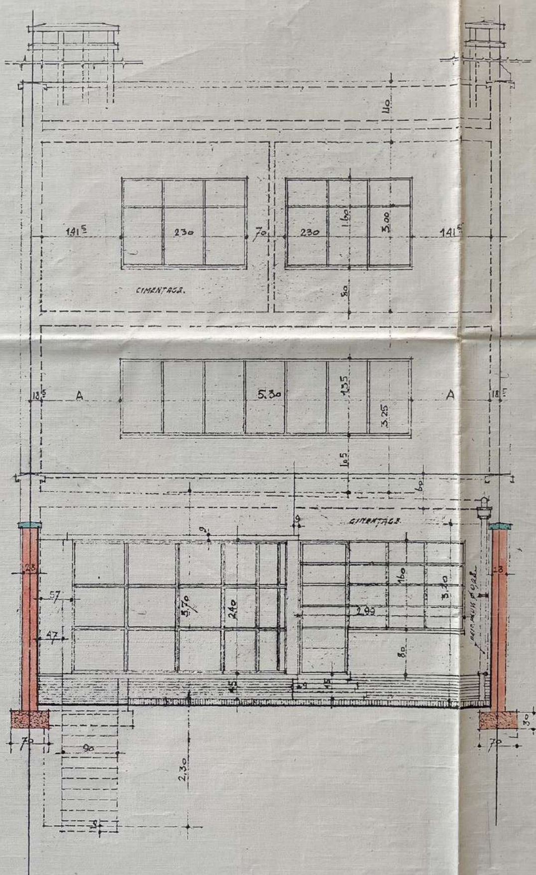
FACADE POSTÉRIEURE,
